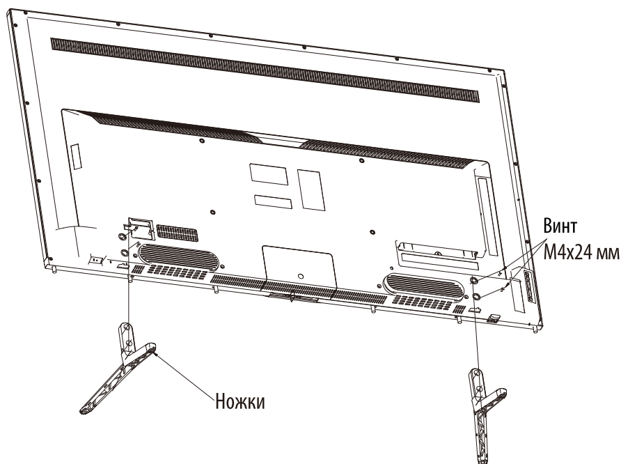
M4x24 мм (4 шт.)
